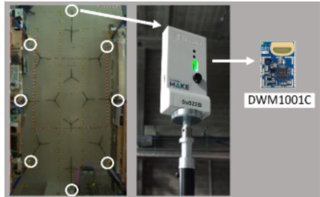
Figure 94: UWB anchor tags
